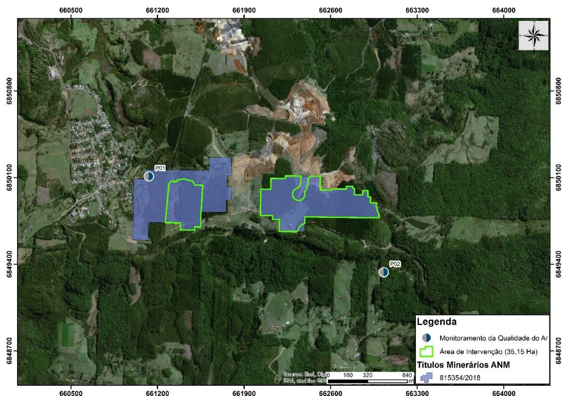
Figura 31: Localização dos pontos de amostragem.
