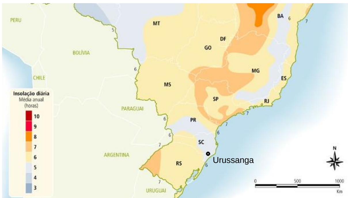
Figura 28: Indicação da insolação diária.
